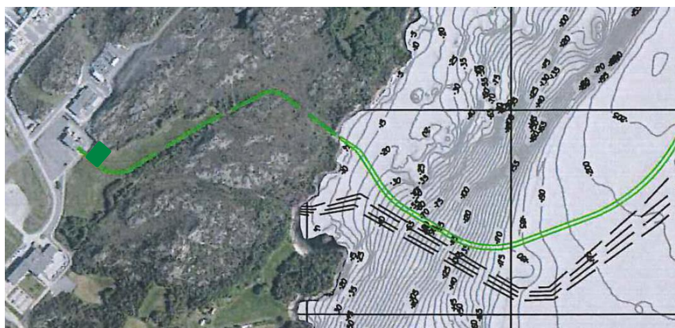
Figur 3-3. Nytt tilegnet område utenfor eksisterende anlegg på Nyhamna (grønn,) ny kabeltrasé og eksisterende kabler i sjø.
